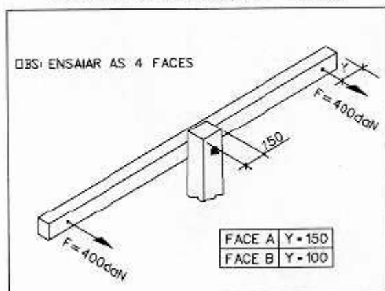
DETALHE PARA ENSAIO DE FLEXÃO
