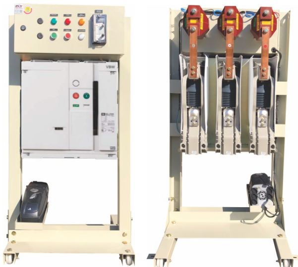
Versão OFFBoard (AxLxP 1.000 x 700 x 600mm)
