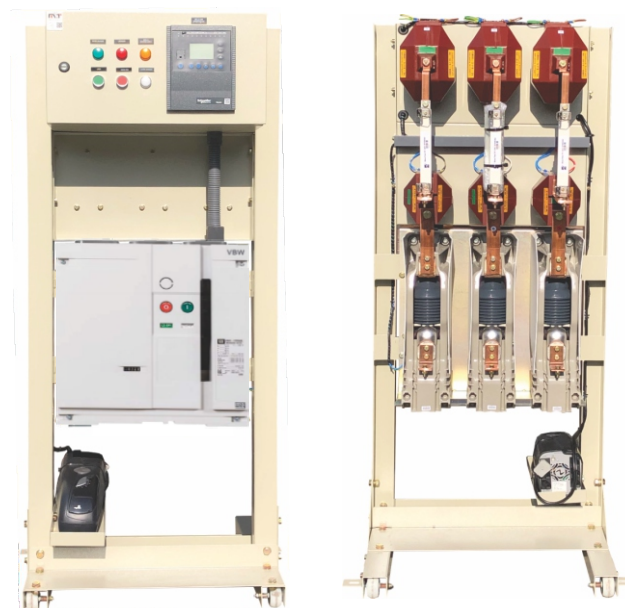
Versão W Solution * (AxLxP 1.400 x 700 x 700mm)
