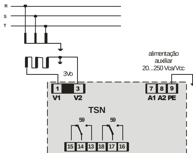
Figura 2: Diagrama de conexão.
